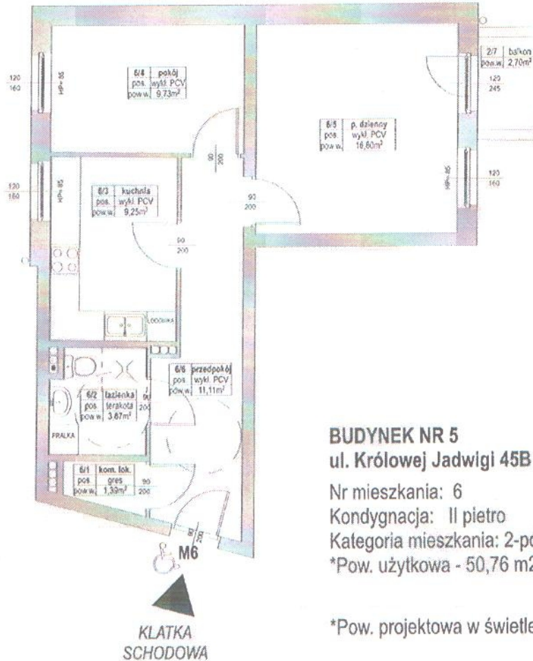
SCHEMAT ROZMIESZCZENIA MIESZKAŃ BUDYNKU NR 5 - II PIĘTRO
